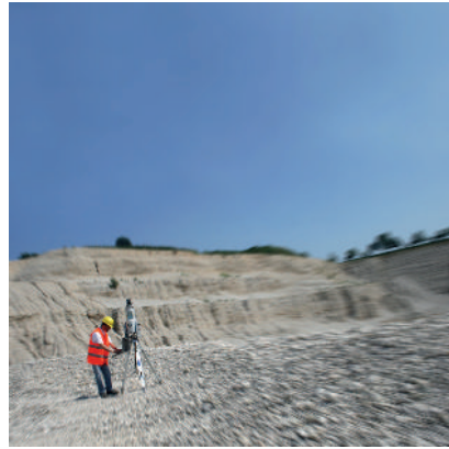
Rilievo di cava con laser scanner 3D
